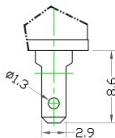
TIPOS DE TERMINAIS DISPONÍVEIS ESC.2:1
