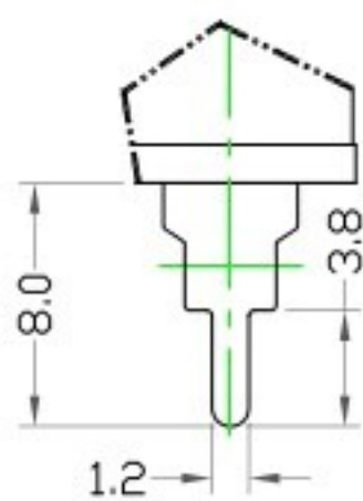
TIPOS DE TERMINAIS DISPONÍVEIS ESC.2:1
